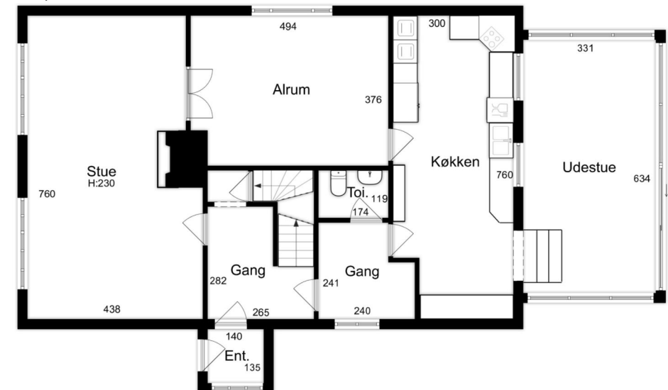
Stueplan
