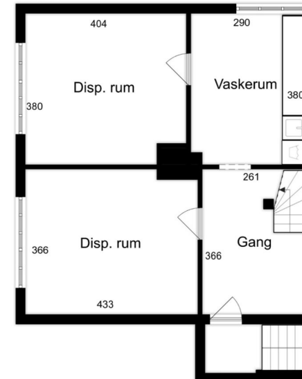
Kælder
