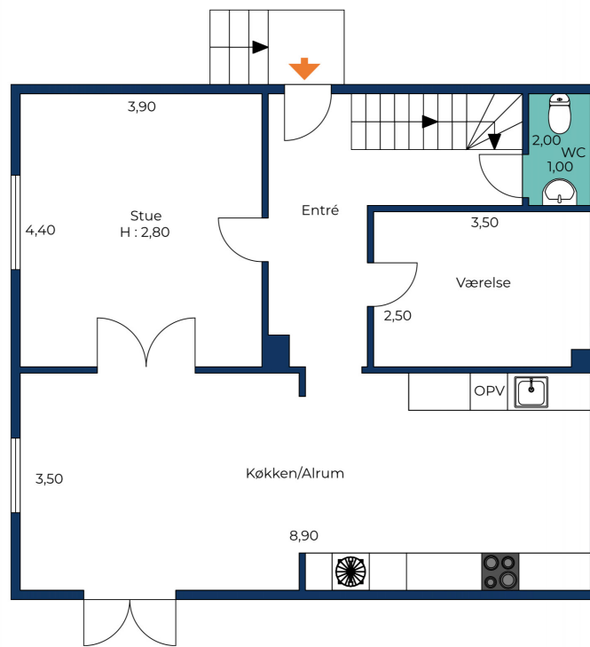
Stueplan
