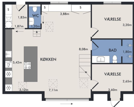
STUEPLAN
