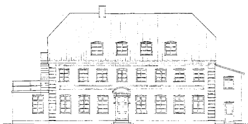
Østfacade eksisterende
