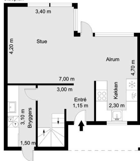
Stueplan
