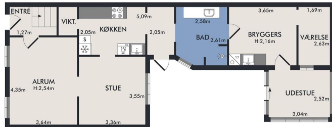
STUEPLAN
