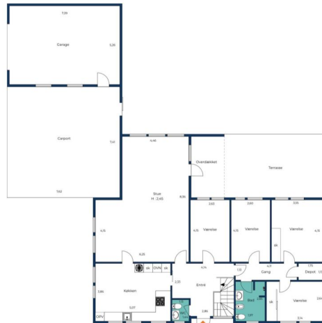
Stueplan
