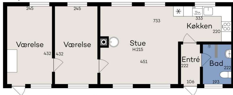
Stueplan
